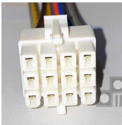
Conector aire acondicionado CA536
