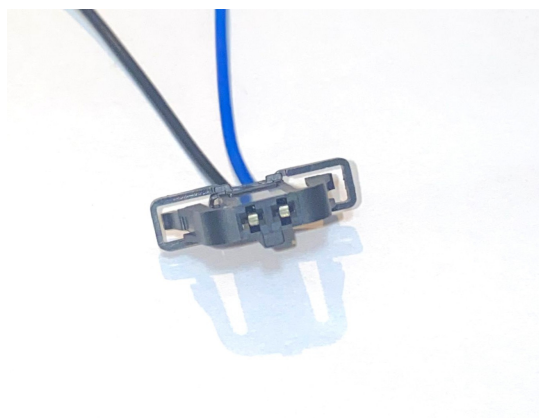
Conector Motor de Control del Actuador de Cerradura de la Puerta del Tanque de Combustible VW
