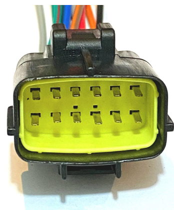
Conector sensor de la caja de cambios, conector hembra hermetico de 12 vias de CA530
