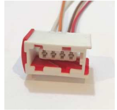
Conector Bosch 4 vias CA299
