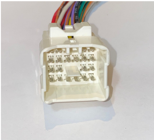
Conector hembra de 20 vias juego de CA572
