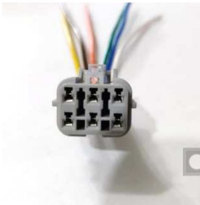
Conector bomba de gasolina Kia rio, Sportage ,Hyundai tucson, Daewoo cielo 95-2003 CA327
