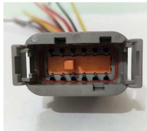
Conector deustch mini 12 vias portamacho
