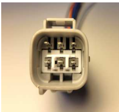
Conector hembra CA 456
