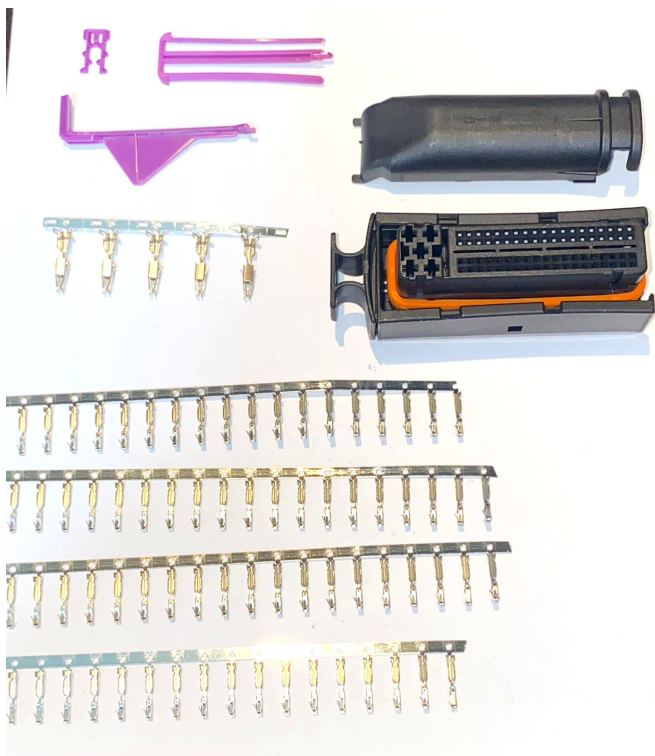
Conector Automotriz ECU de 81 Vías Gimax, Tyco 1J0906385C / 1J0 906 385C / 368376-1 / 368389-1 / 368382-1, VW/Audi/SEAT/Skoda CA539
