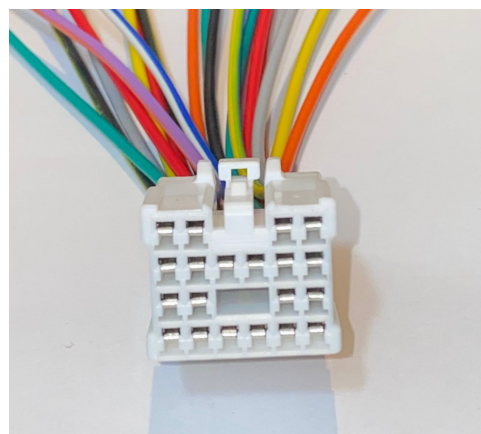
Conector macho de 20 vías juego de CA573
