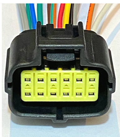
Conector sensor de la caja de cambios, conector macho hermetico de 12 vias CA530
