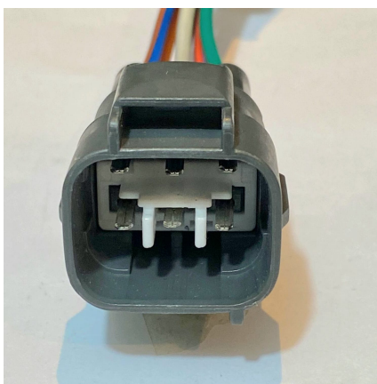
Conector hembra de CA456, luces y motor Toyota
