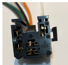
Conector del pedal del acelerador, sensor MAF, Toyota y Mazda. CA541
