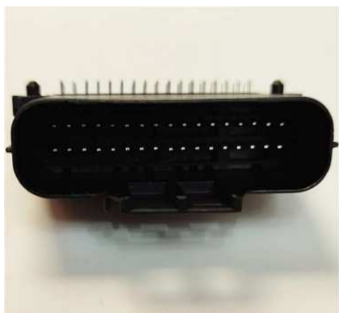
Conector 34 vias de chasis porta macho compañero CA363
