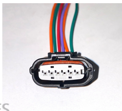
Conector del pedal del acelerador, sensor MAF, Toyota y Mazda. CA541
