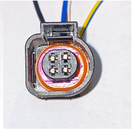
Conector Sensor Temperatura Skoda Volkswagen
