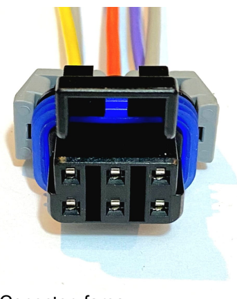
Conector faros, Direccionales GMC, GM, CADILLAC
