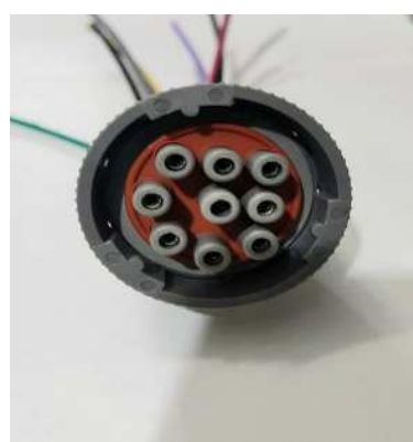
Conector deutsch 9 pin diagnostico obd2 maquinaria, varios hyundai compañero de CA430
