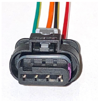
Conector luz trasera, Sensor de posición del árbol de levas OEM 05149141AF VW PC950 Compatible con Jeep Dodge Ram Chrysler Hyundai Volkswagen CA534
