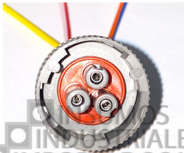
Amp HD16-3-16S conector 3 contactos hembra HD10 CA550
