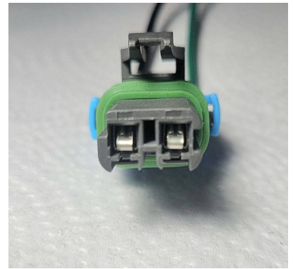
Conector regulador de motor GM (Dorman 645-200)
