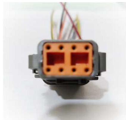
Conector deustch mini 8 vias portahembra
