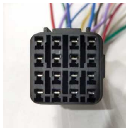
Conector portahembra 16 vias para aire acondicionado compañero de CA337
