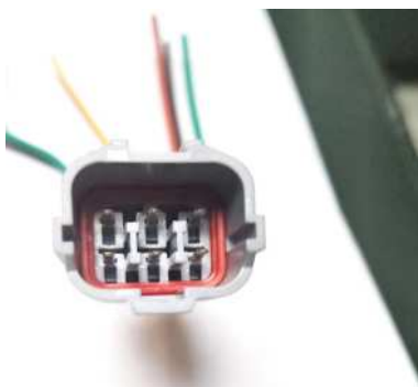
Conector 6 vias hembra compañero CA327
